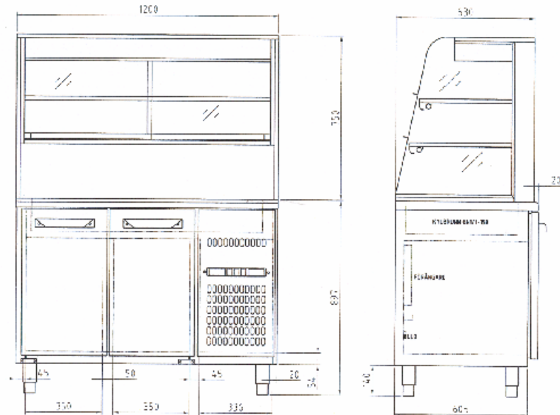
Kylmonter DEM 1200 – 2 med kylbänk ABTF 1200
